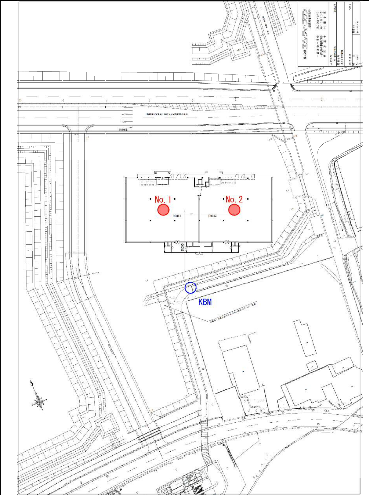
ボーリング調査位図
